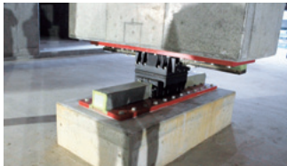
転がりリローラー支承
